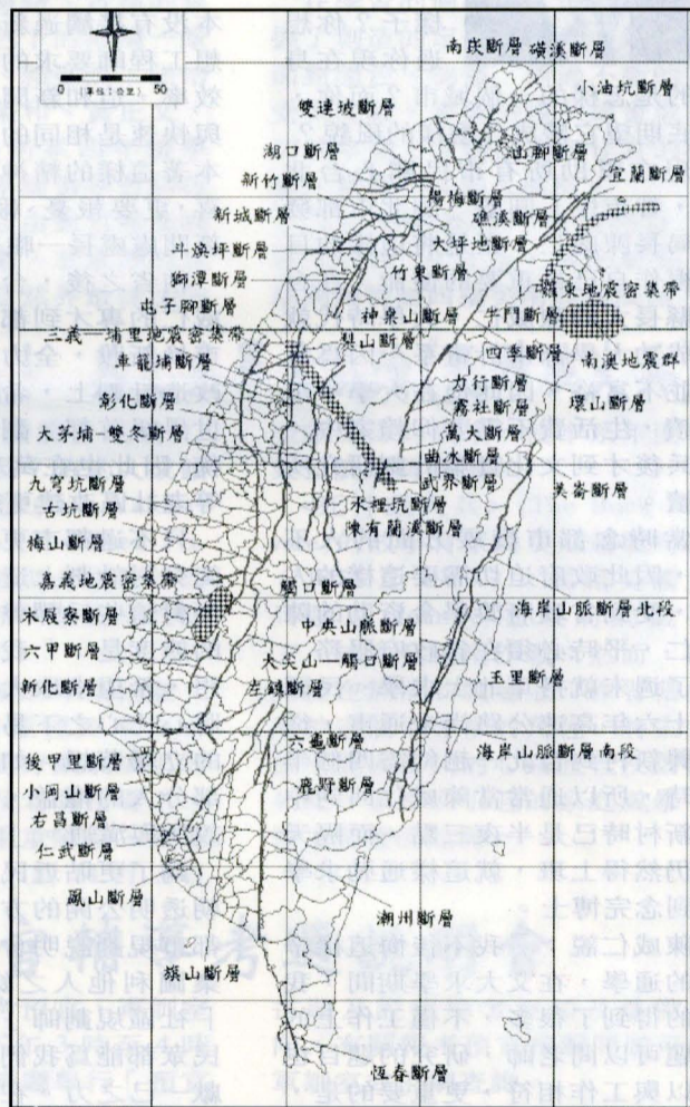
臺灣地區活斷層分佈圖
