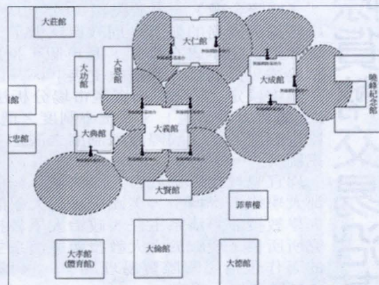
無線網路室外涵蓋範圍圖。
