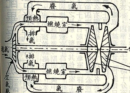
汽車用氣體渦輪機之構造原理
