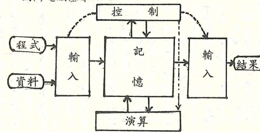
圖(b)--->控制訊號流向->資料流向
