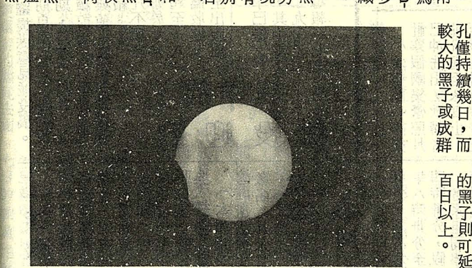
日偏蝕直焦攝影，圖中黑點部分為太陽黑子。
