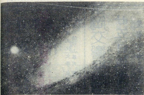
• 仙女座大星雲 M31
