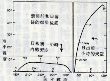
圖二：北緯40度內可見之奧斯汀彗星的地平經度和地平緯度。由圖可知4月20日後奧斯汀升至仰角較高處，因此較易觀測。
