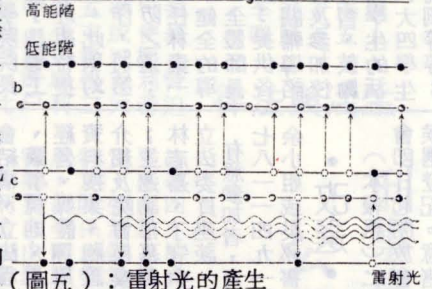
(圖五)：雷射光的產生 (a)雷射介質在熱平衡時之粒子能階分布情形 (b)雷射介質在受到起能後，處於反常分布情況下 (c)由一個自衰變的粒子發出的光子經不斷的加強及偶而的減弱而生成強大的雷射光。
