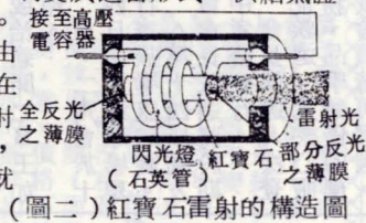
(圖二) 紅寶石雷射的構造圖
