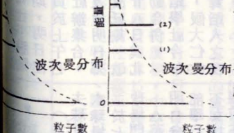
(圖四) 「粒子」能階的分布情形比較。
